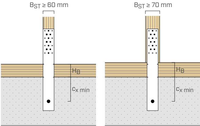
10 elemente de fixare LBA Ø4 x 60
