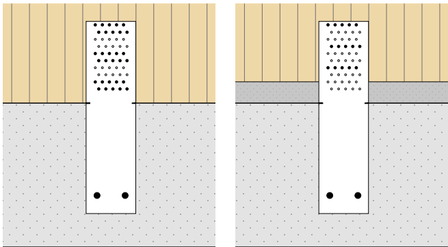
30 elemente de fixare fixare parțială LBA Ø4 x 60 | SBS Ø5 x 60
