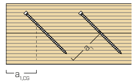
Aufriss
