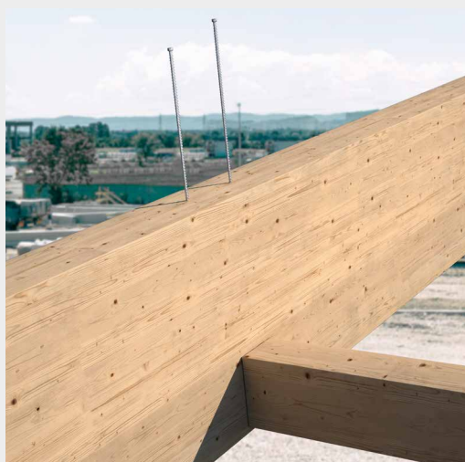
^ Renfort orthogonal par rapport à la fibre pour charge suspendue due à l'assemblage poutre principale – secondaire.
