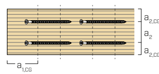
Draufsicht
