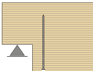
Querschnitt
