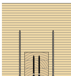
nárys
