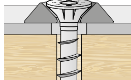
Κυλινδρική οπή με λιμαρισμένη ροδέλα HUS.
